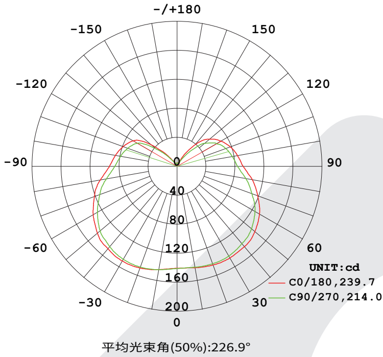
配光曲线
